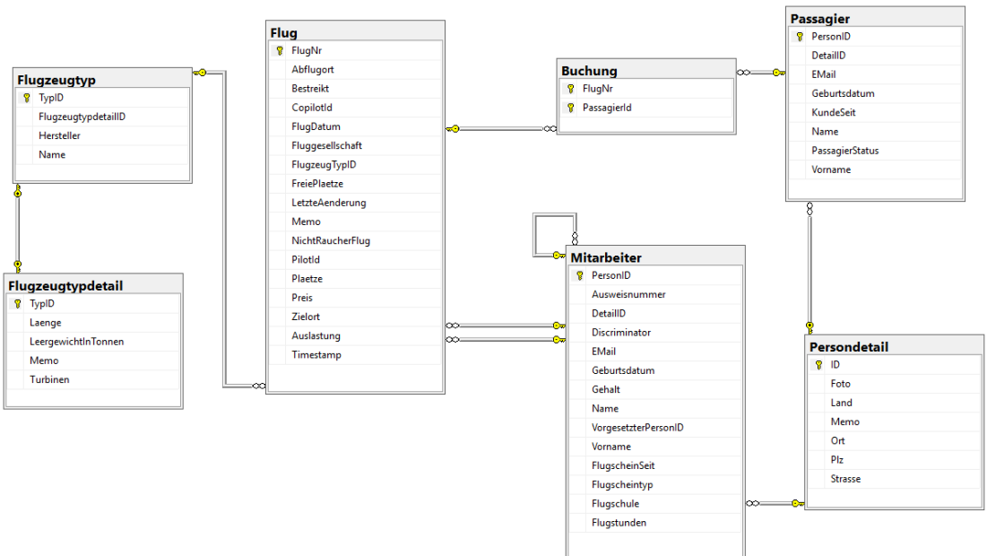
Bild 1.4 World Wide Wings-Datenmodell in der komplexeren Version
