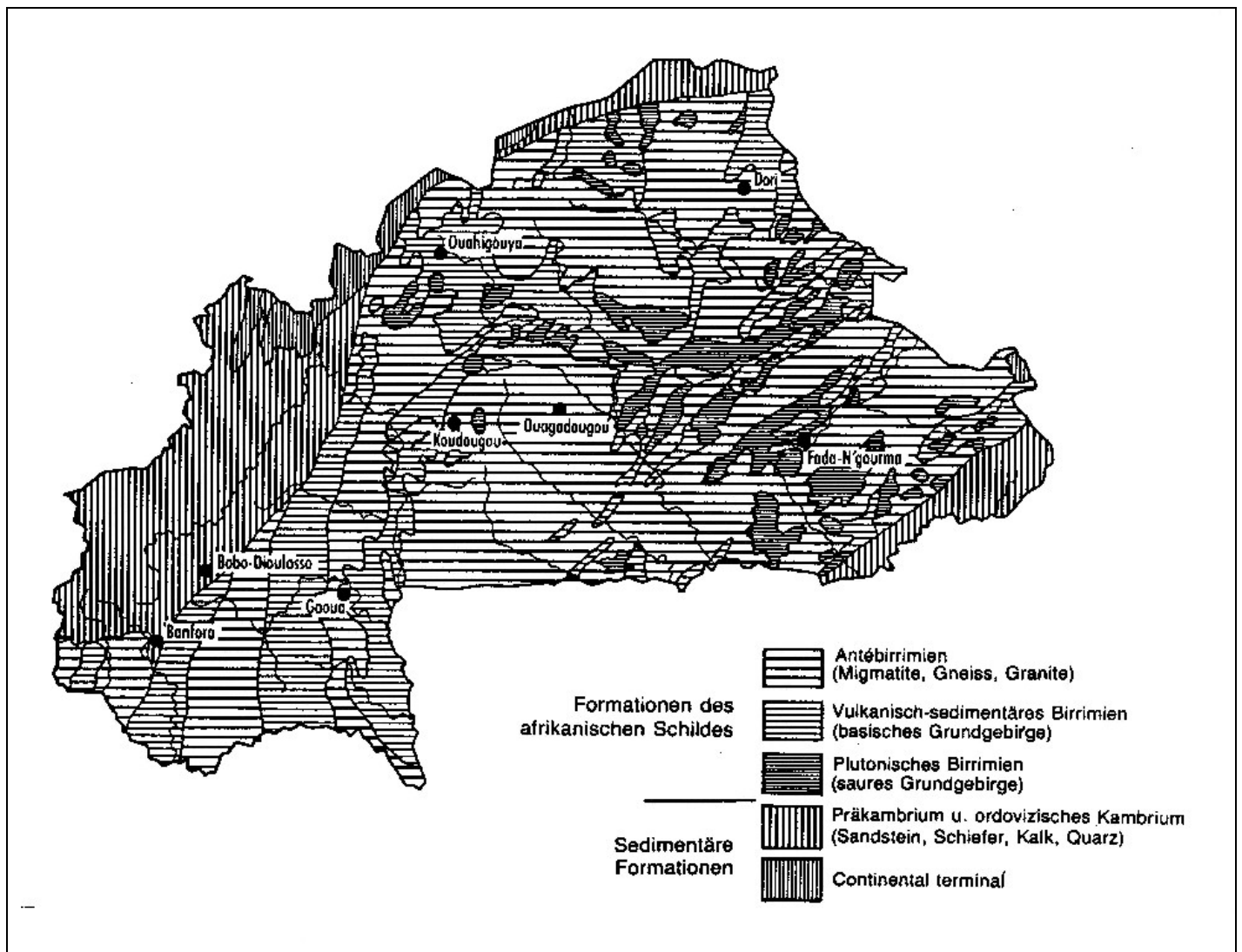
Abb. 2: Geologische Karte von Burkina Faso
